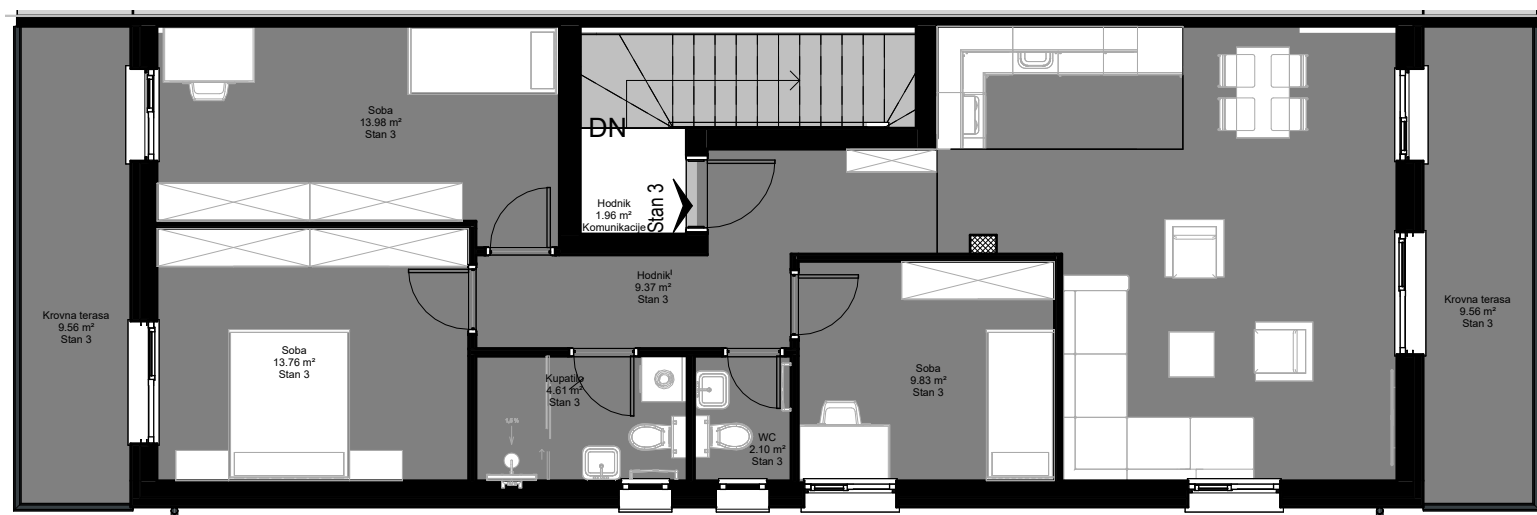
1 C02 - Potkrovlje - Položaj stana 3 na osnovi 1 : 100
