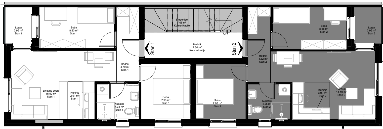
1 C02 - Sprat - Položaj stana 2 na osnovi 1 : 100
